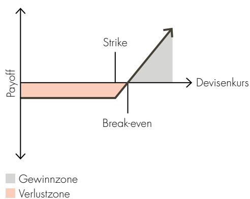
Payoff-Diagramm für Long-Call-Option
