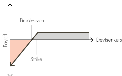
Payoff-Diagramm für Short-Put-Option
