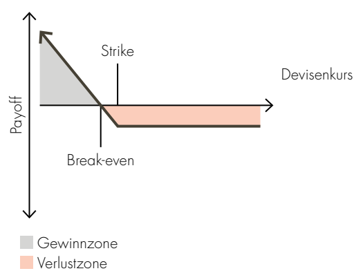
Payoff-Diagramm für Long-Put-Option
