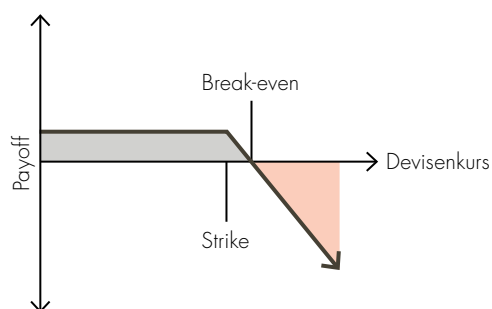
Payoff-Diagramm für Short-Call-Option
